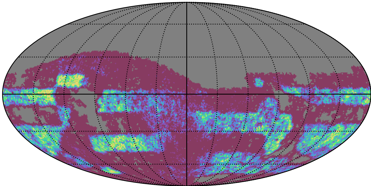
no_long_daily_v3.4_10yrs Yr 3-4 g band: NVisits
