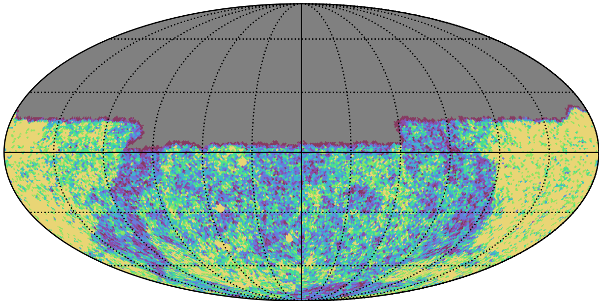
no_long_daily_v3.4_10yrs Yr 1 u band: NVisits
