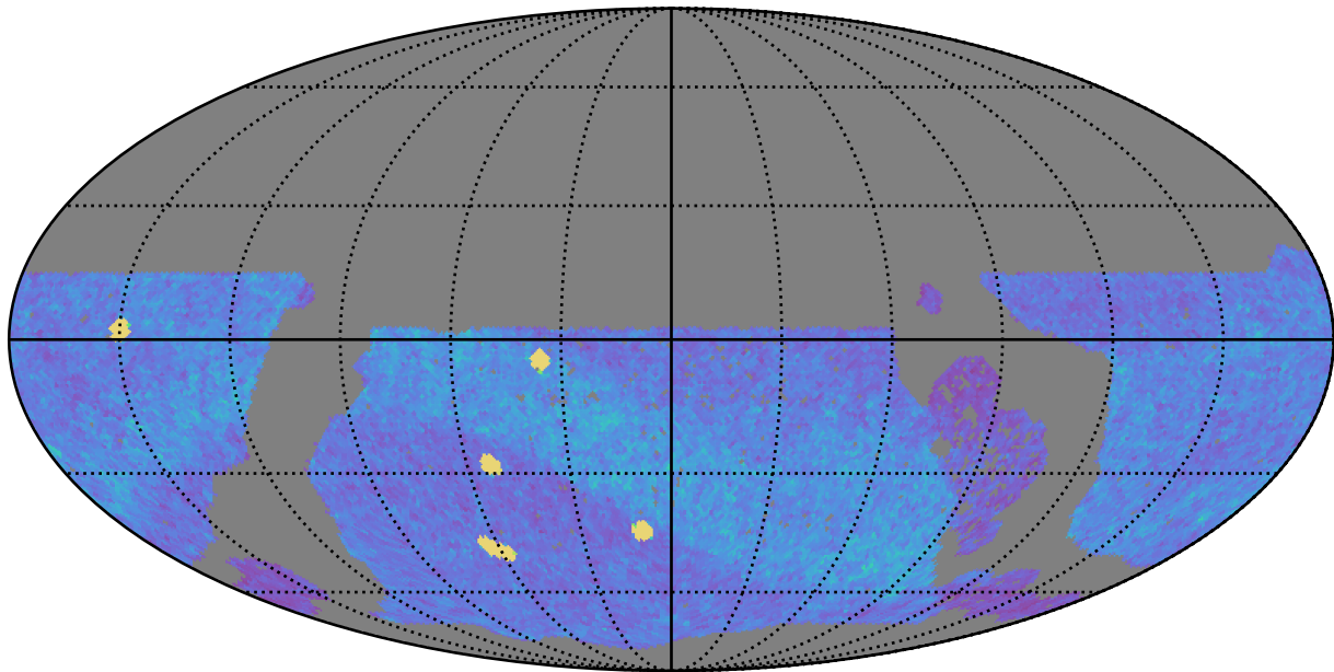
no_long_daily_v3.4_10yrs WFD z band: NVisits
