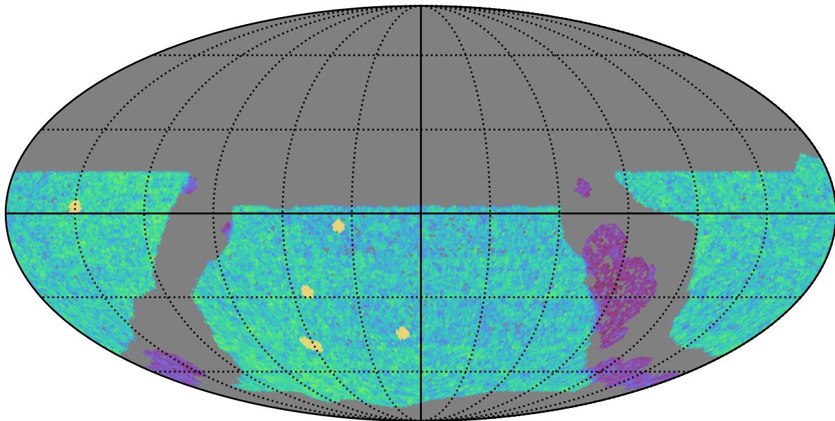
no_long_daily_v3.4_10yrs WFD u band: NVisits
