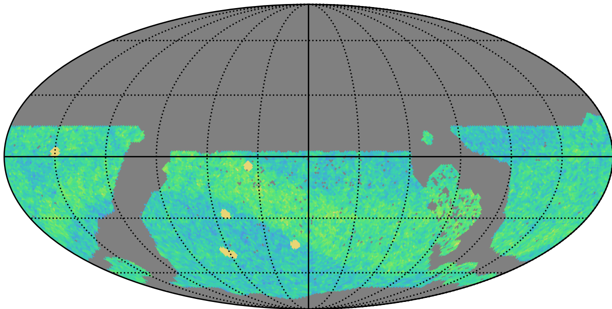
no_long_daily_v3.4_10yrs WFD i band: NVisits
