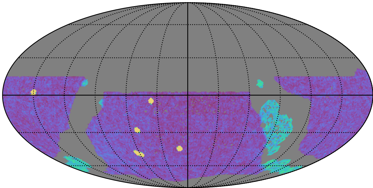
no_long_daily_v3.4_10yrs WFD g band: NVisits
