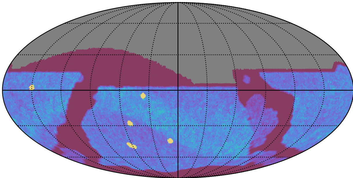
no_long_daily_v3.4_10yrs All sky z band: NVisits
