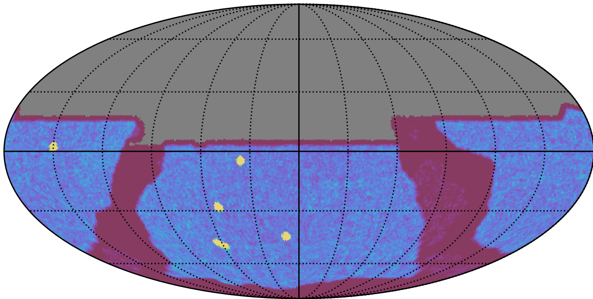
no_long_daily_v3.4_10yrs All sky y band: NVisits
