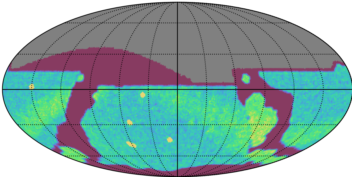
no_long_daily_v3.4_10yrs All sky r band: NVisits
