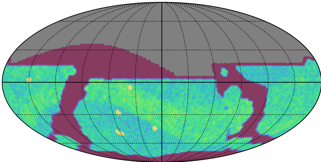
no_long_daily_v3.4_10yrs All sky i band: NVisits
