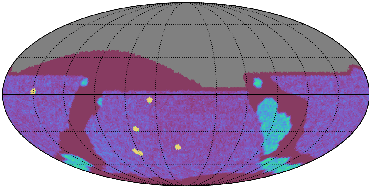
no_long_daily_v3.4_10yrs All sky g band: NVisits
