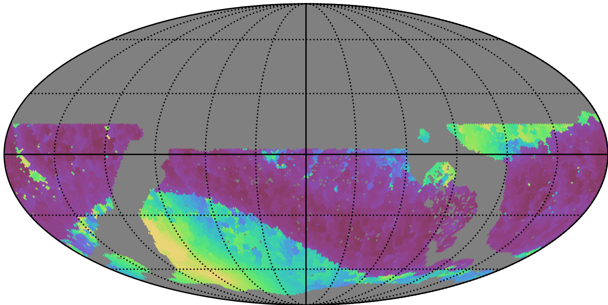
no_long_daily_v3.4_10yrs WFD z band: Min solarElong
