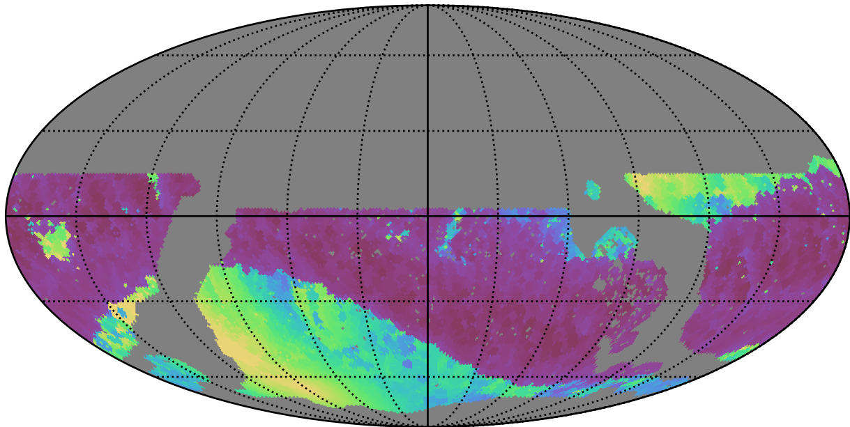
no_long_daily_v3.4_10yrs WFD i band: Min solarElong
