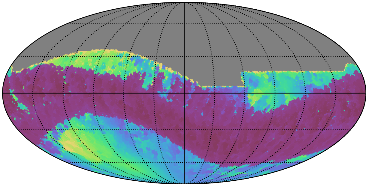
no_long_daily_v3.4_10yrs All sky z band: Min solarElong
