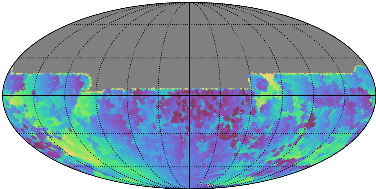
no_long_daily_v3.4_10yrs All sky y band: Min solarElong
