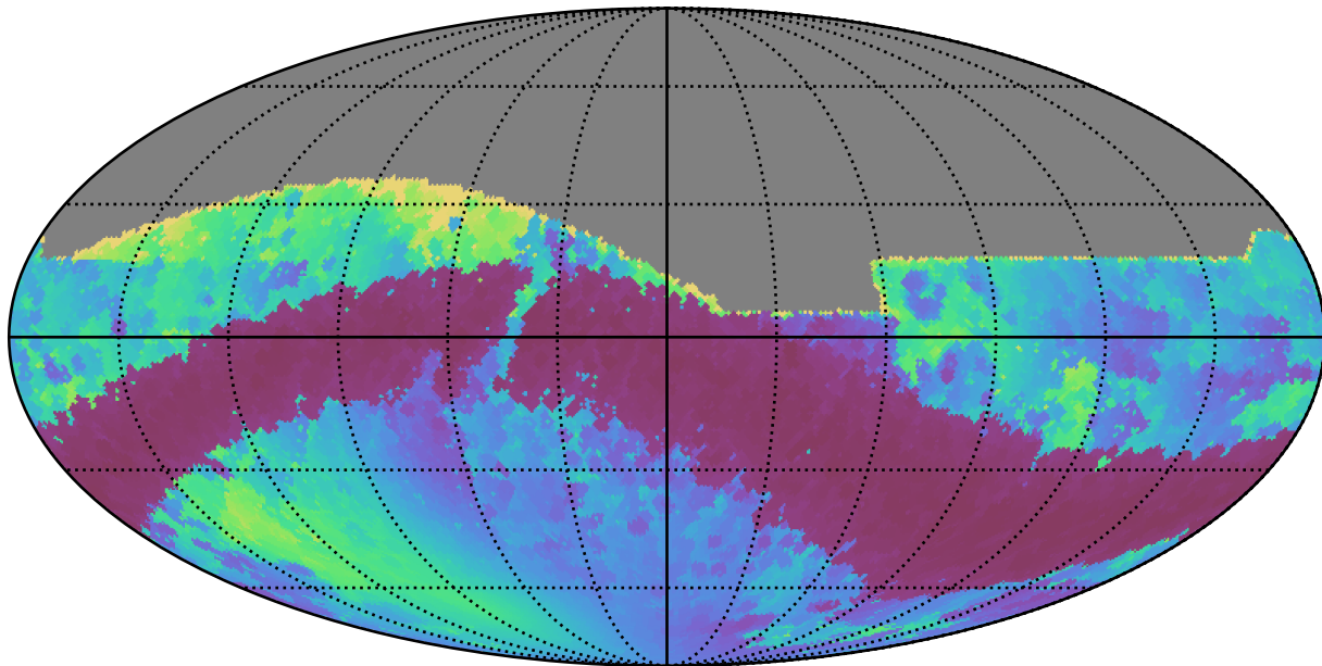
no_long_daily_v3.4_10yrs All sky r band: Min solarElong
