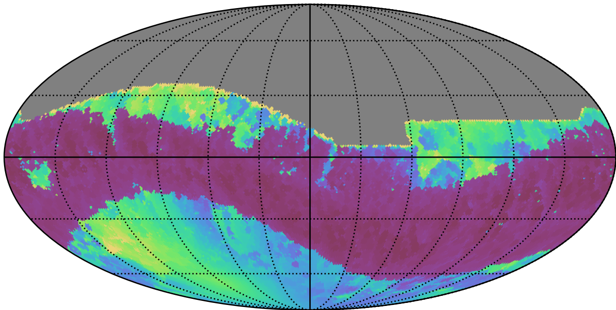
no_long_daily_v3.4_10yrs All sky i band: Min solarElong
