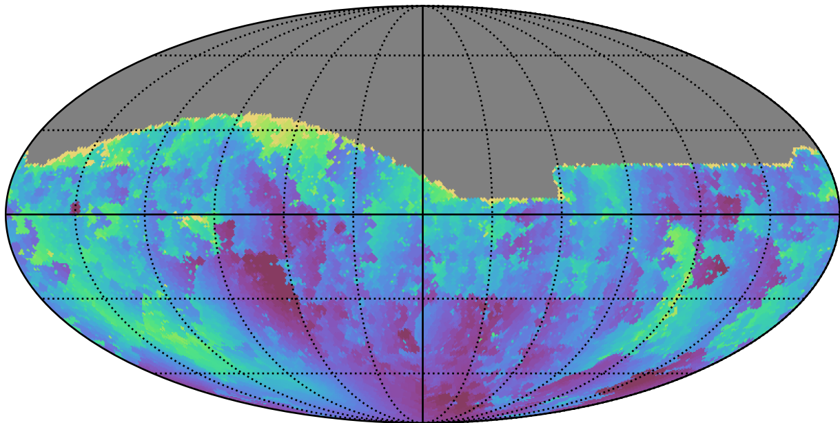
no_long_daily_v3.4_10yrs All sky g band: Min solarElong
