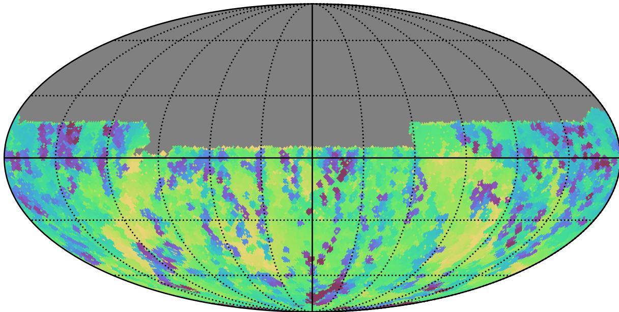
no_long_daily_v3.4_10yrs Yr 1 y band: Min skyBrightness
