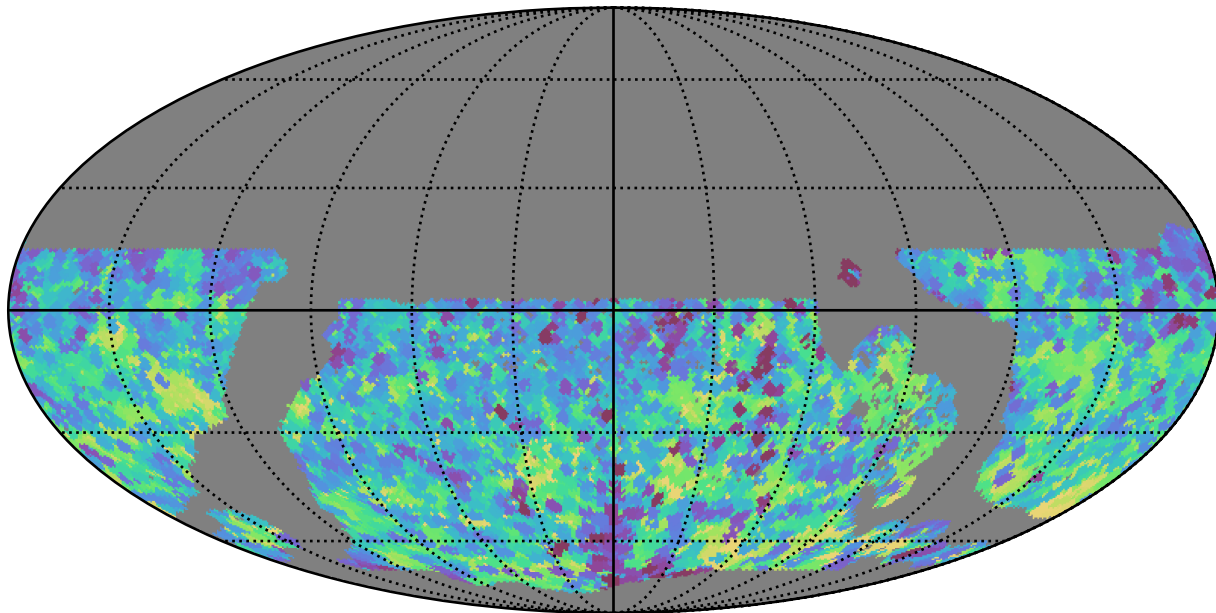
no_long_daily_v3.4_10yrs WFD y band: Min skyBrightness
