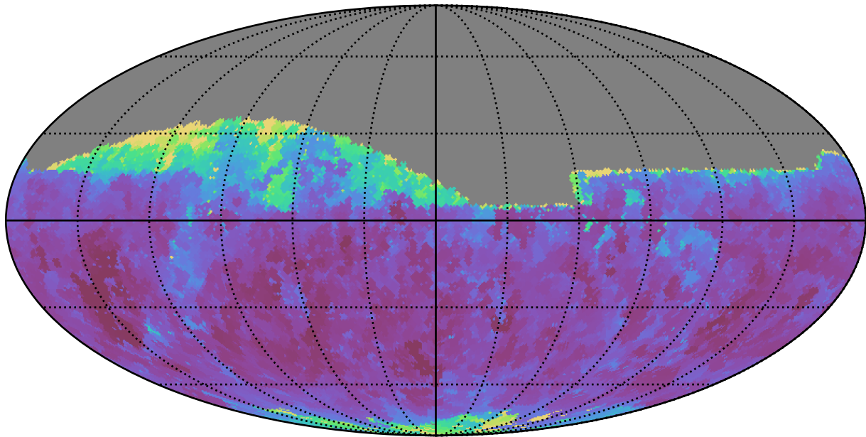
no_long_daily_v3.4_10yrs Yr 1 i band: Min seeingGeom
