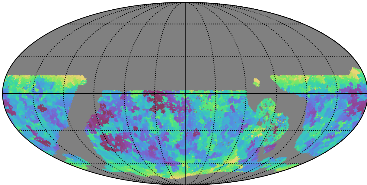
no_long_daily_v3.4_10yrs WFD y band: Min seeingEff
