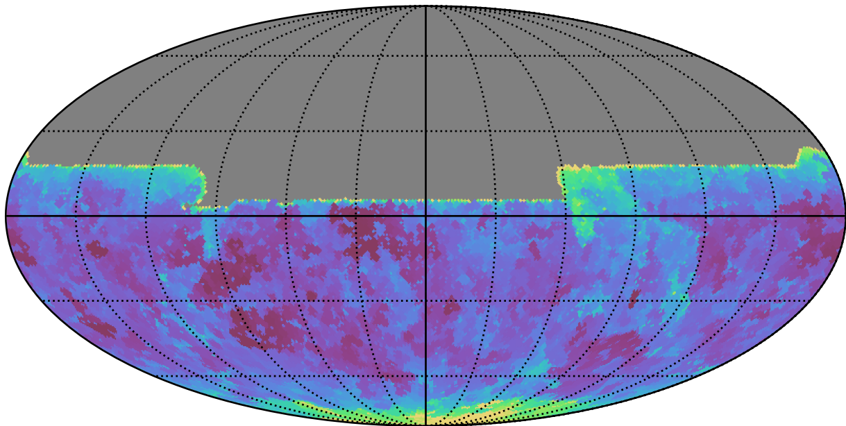
no_long_daily_v3.4_10yrs All sky y band: Min seeingEff
