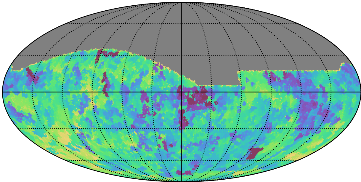
no_long_daily_v3.4_10yrs All sky z band: Min saturation_mag
