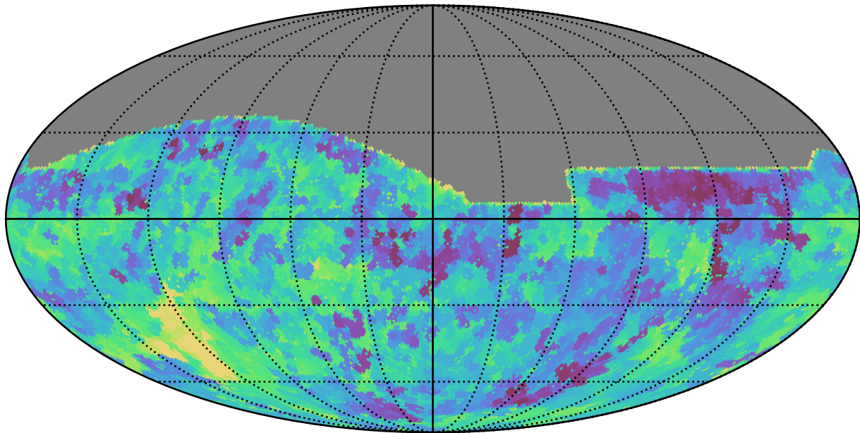
no_long_daily_v3.4_10yrs All sky r band: Min saturation_mag
