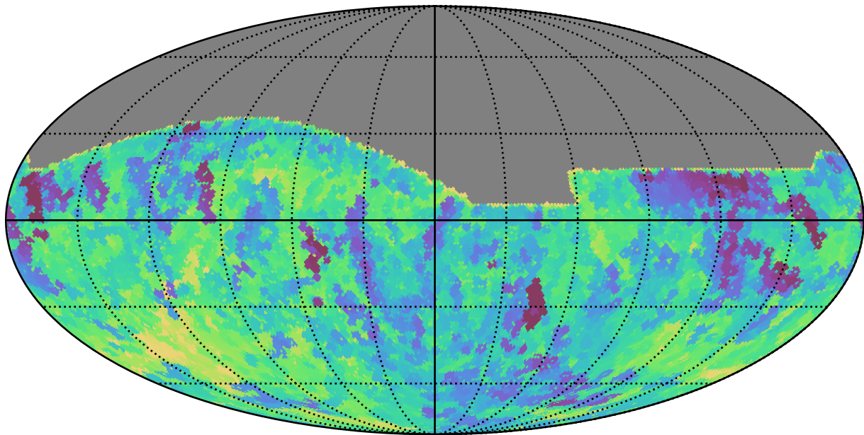
no_long_daily_v3.4_10yrs All sky i band: Min saturation_mag
