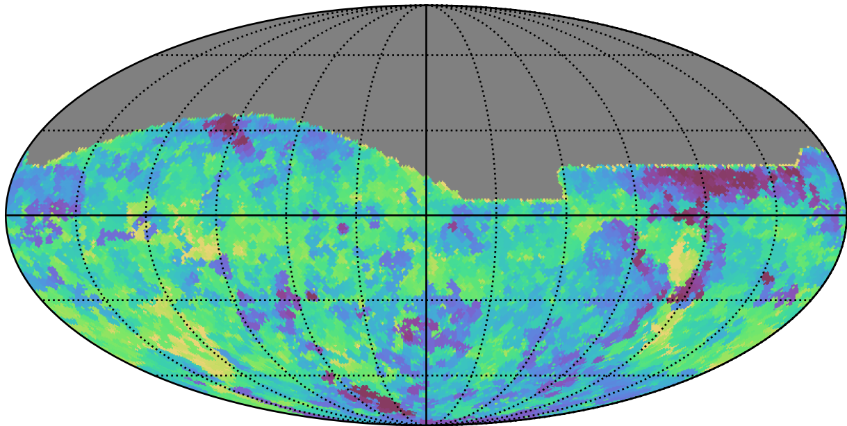
no_long_daily_v3.4_10yrs All sky g band: Min saturation_mag
