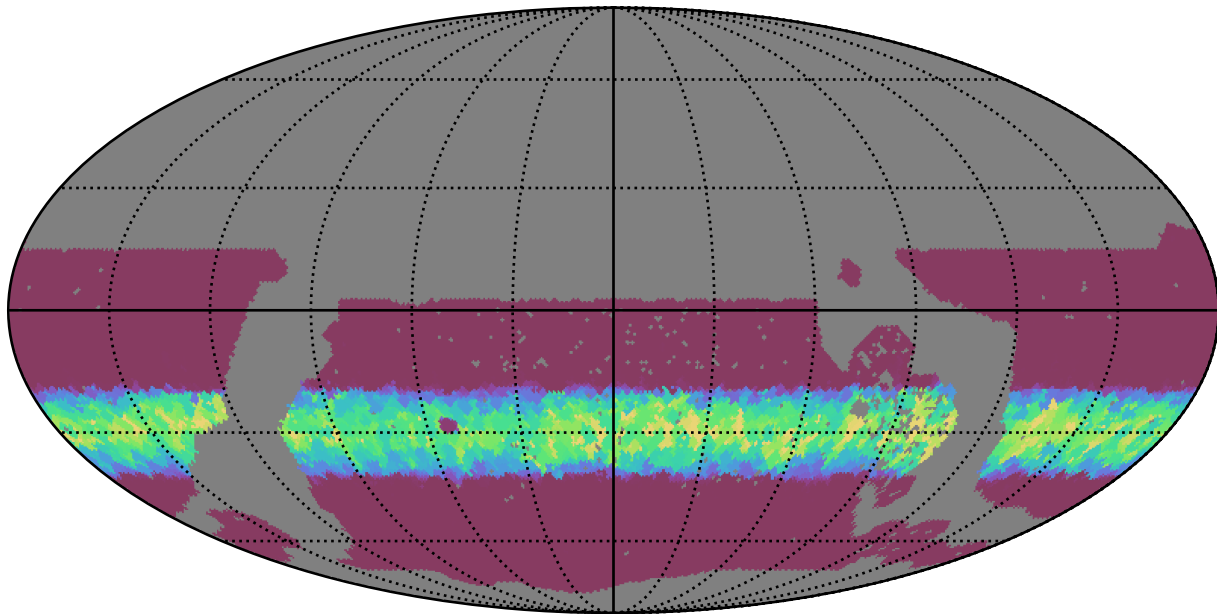
no_long_daily_v3.4_10yrs WFD y band: Min normairmass
