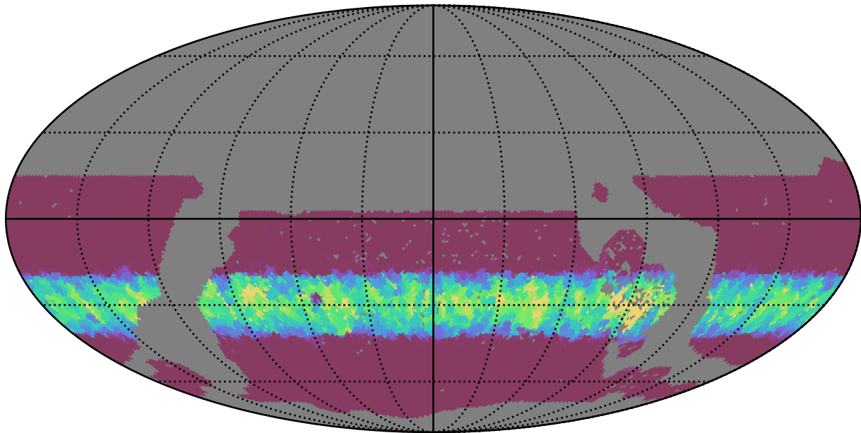
no_long_daily_v3.4_10yrs WFD u band: Min normairmass
