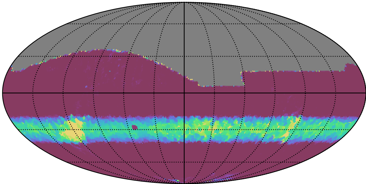
no_long_daily_v3.4_10yrs All sky z band: Min normairmass
