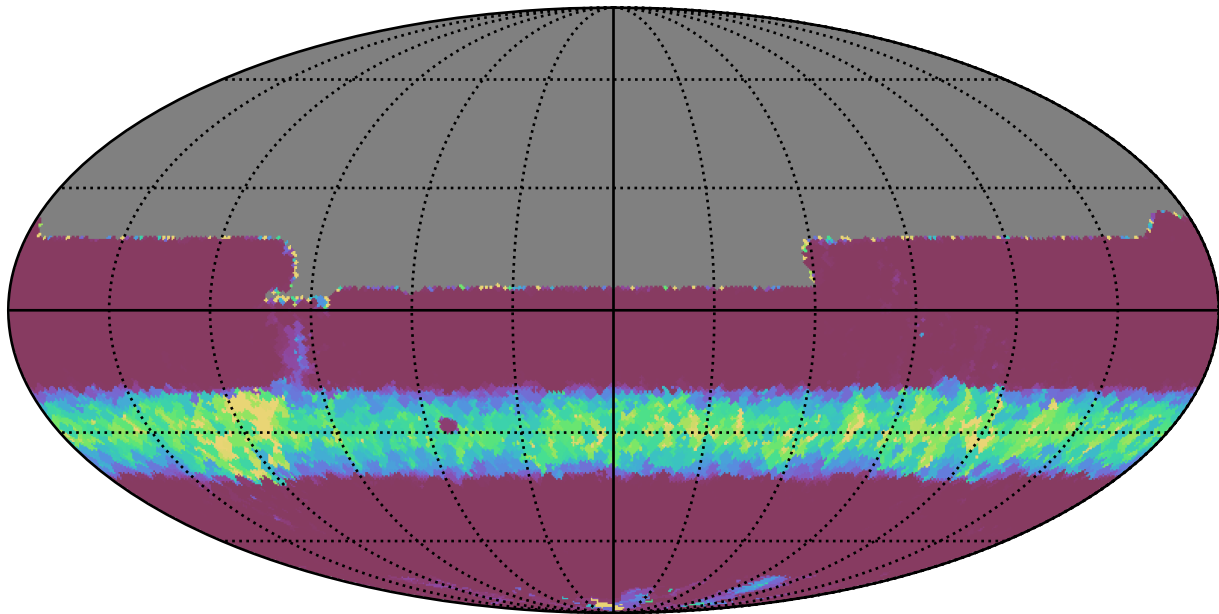
no_long_daily_v3.4_10yrs All sky y band: Min normairmass
