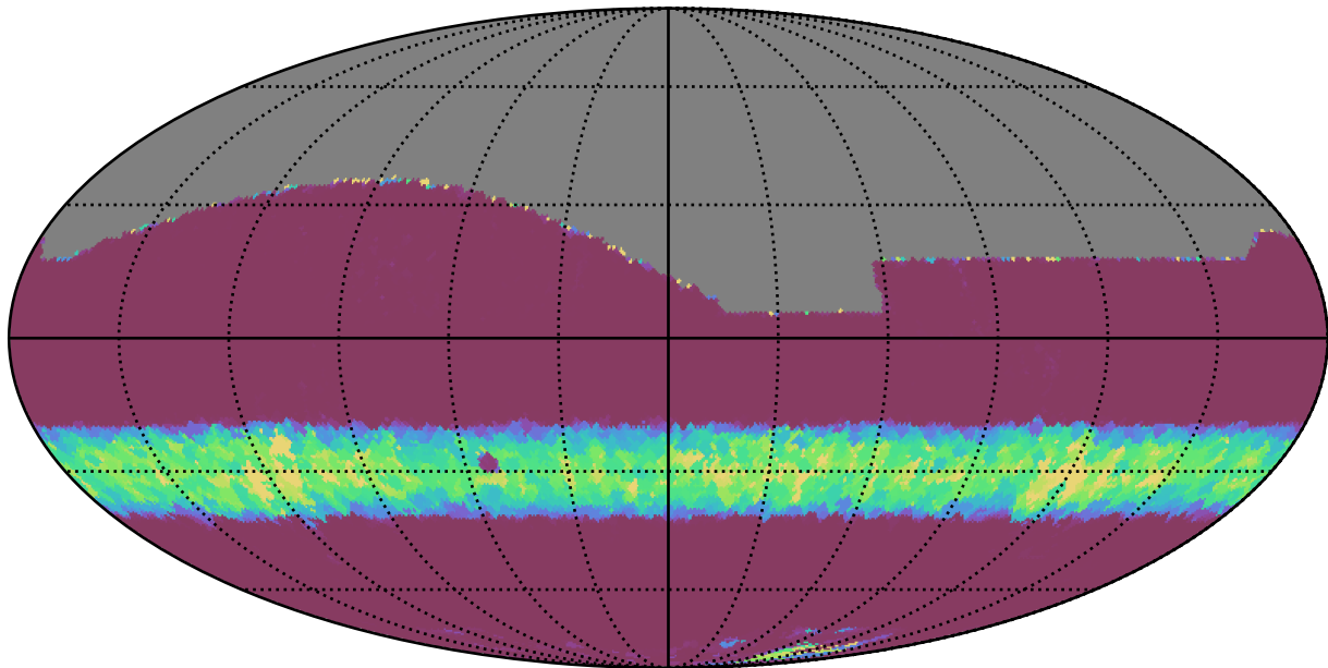
no_long_daily_v3.4_10yrs All sky r band: Min normairmass
