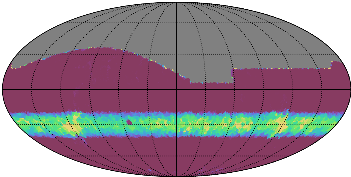
no_long_daily_v3.4_10yrs All sky i band: Min normairmass
