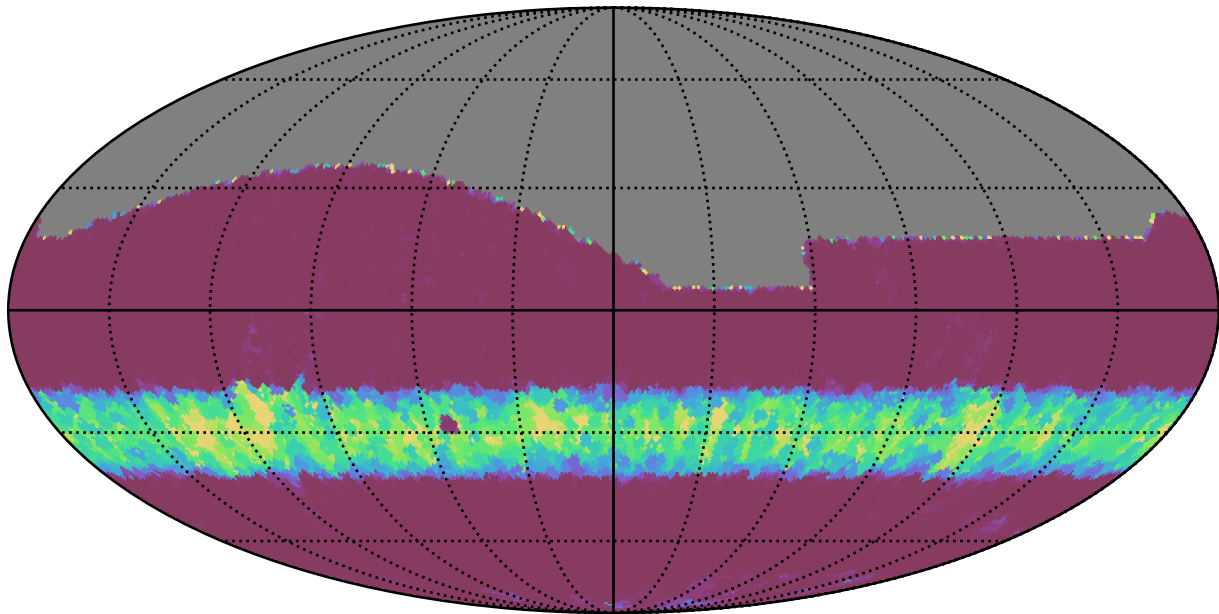
no_long_daily_v3.4_10yrs All sky g band: Min normairmass
