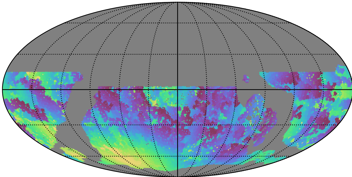
no_long_daily_v3.4_10yrs WFD u band: Min moonDistance
