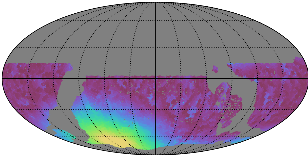
no_long_daily_v3.4_10yrs WFD r band: Min moonDistance
