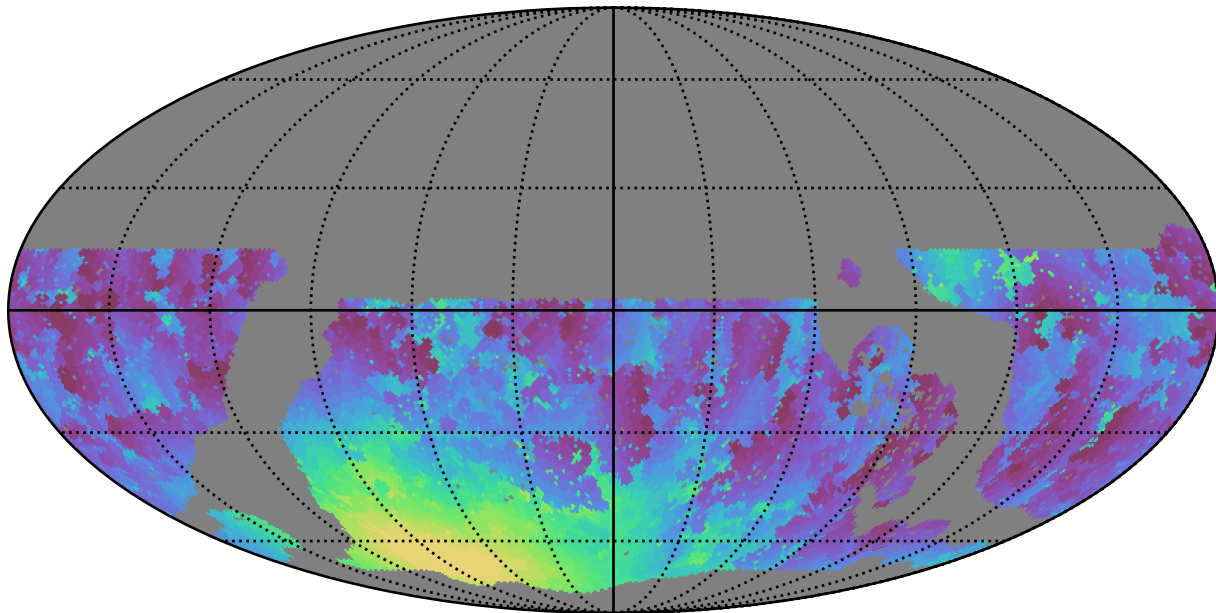
no_long_daily_v3.4_10yrs WFD g band: Min moonDistance
