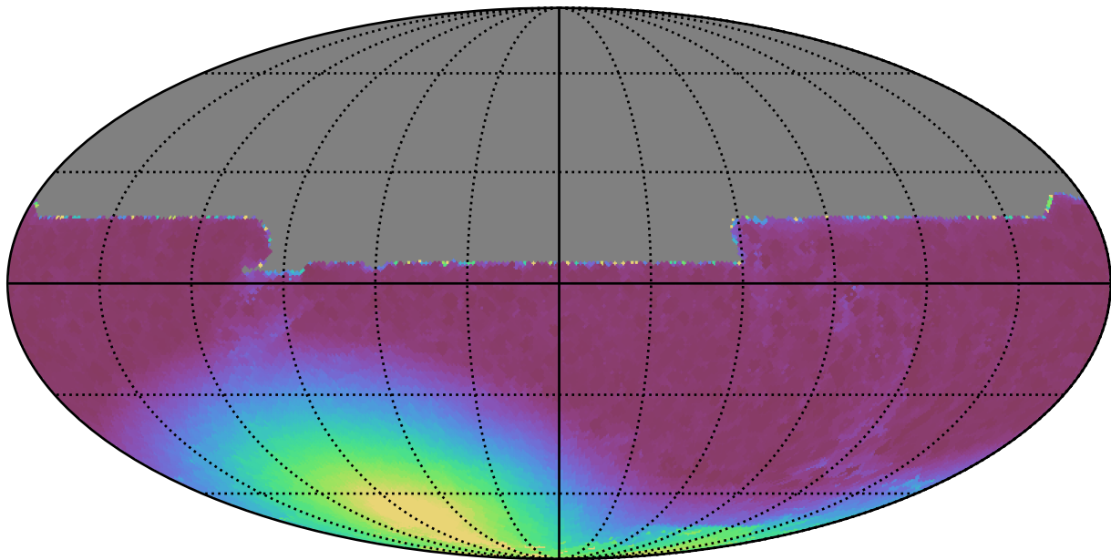
no_long_daily_v3.4_10yrs All sky y band: Min moonDistance
