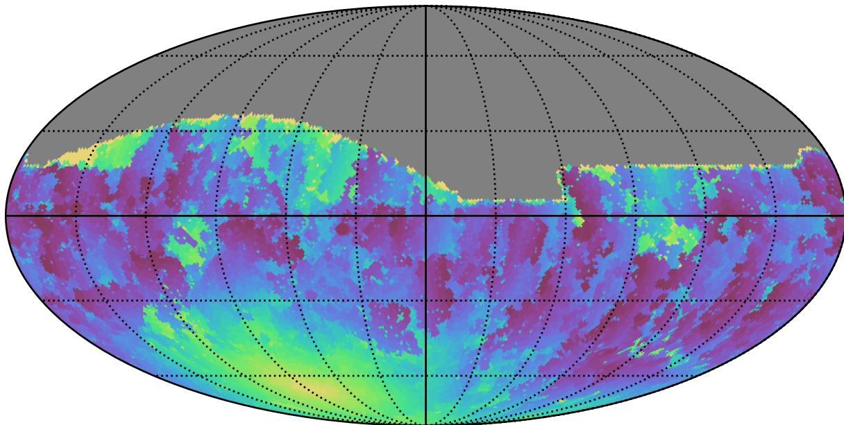
no_long_daily_v3.4_10yrs All sky g band: Min moonDistance
