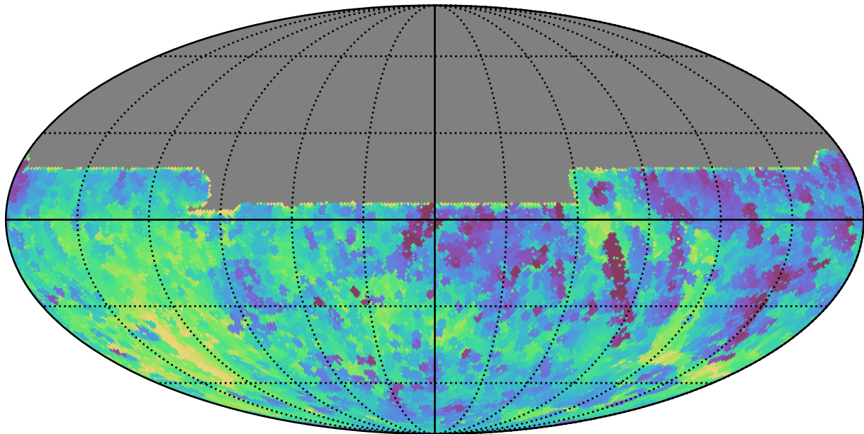
no_long_daily_v3.4_10yrs All sky y band: Min fiveSigmaDepth
