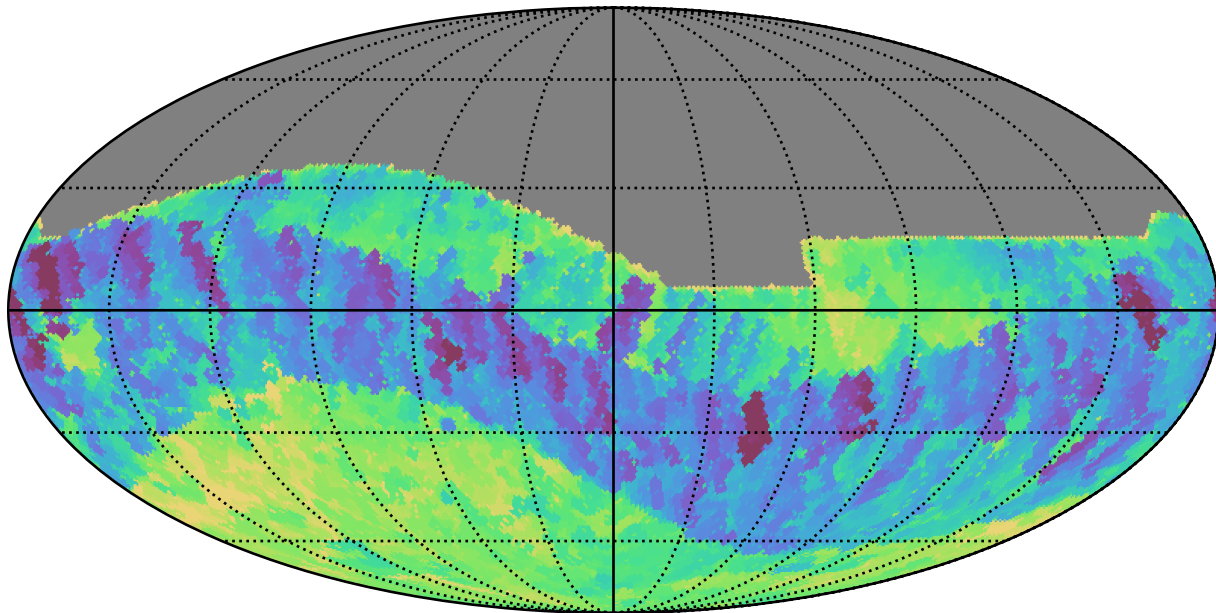
no_long_daily_v3.4_10yrs All sky i band: Min fiveSigmaDepth
