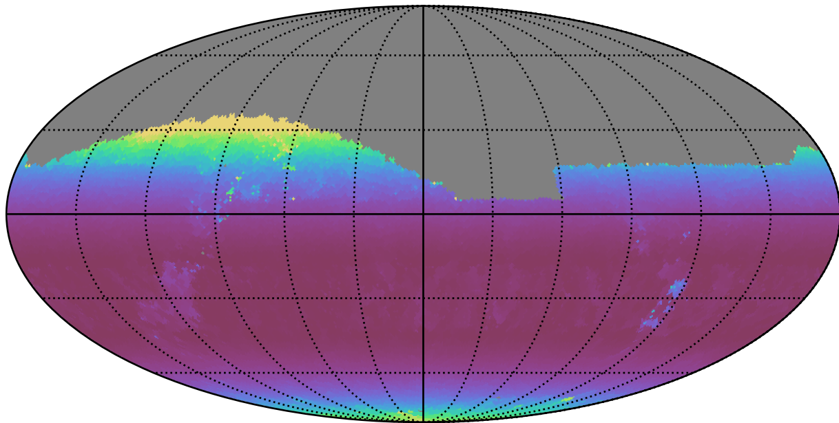
no_long_daily_v3.4_10yrs Yr 1 z band: Min airmass
