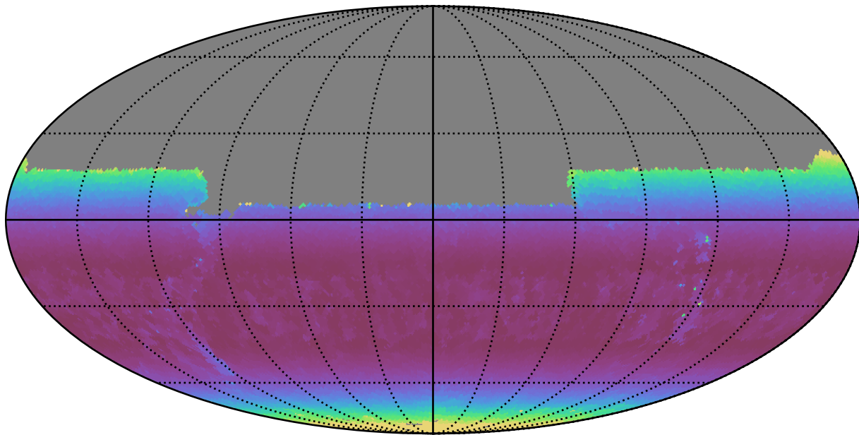
no_long_daily_v3.4_10yrs Yr 1 y band: Min airmass
