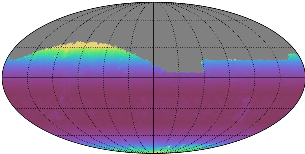
no_long_daily_v3.4_10yrs Yr 1 r band: Min airmass
