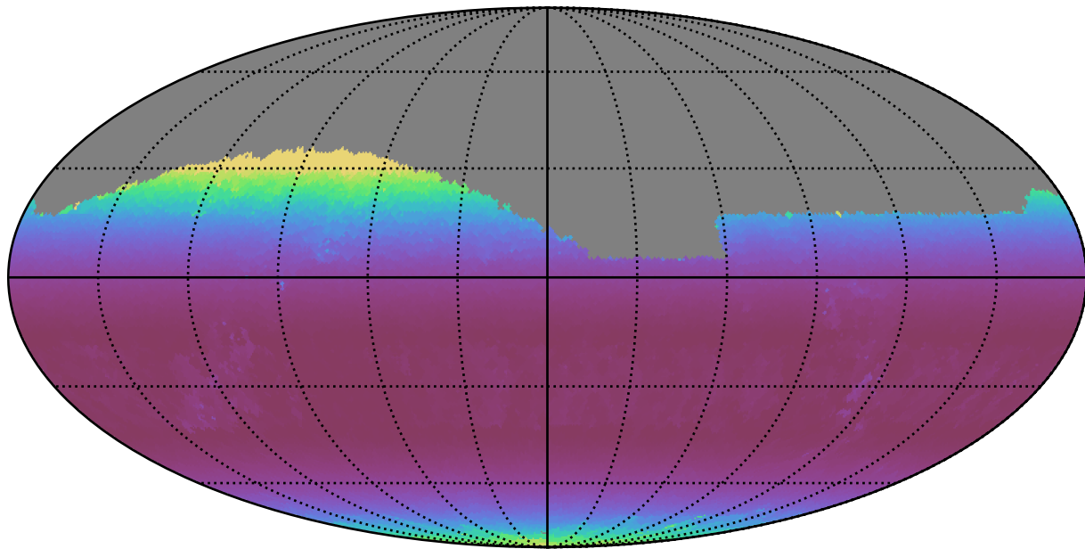
no_long_daily_v3.4_10yrs Yr 1 i band: Min airmass
