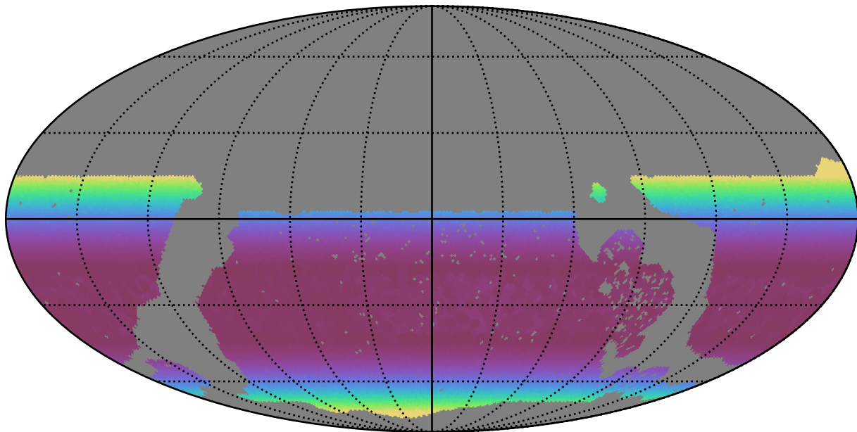
no_long_daily_v3.4_10yrs WFD z band: Min airmass
