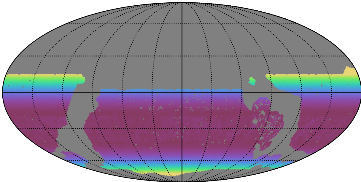
no_long_daily_v3.4_10yrs WFD y band: Min airmass
