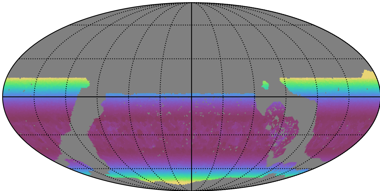
no_long_daily_v3.4_10yrs WFD u band: Min airmass
