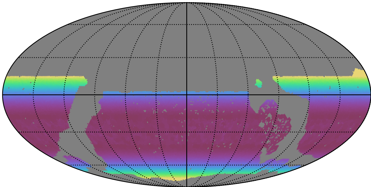
no_long_daily_v3.4_10yrs WFD r band: Min airmass
