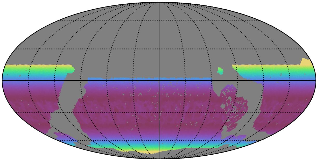
no_long_daily_v3.4_10yrs WFD g band: Min airmass
